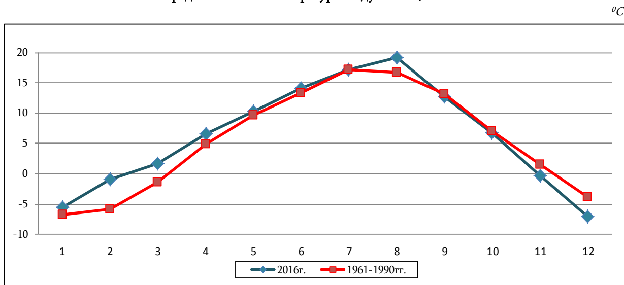
Среднемесячная температура воздуха в РА, 2016г.
